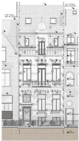
Façade avant Projetée
