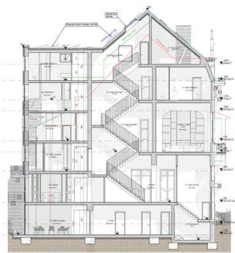
Coupe A-A Projetée
