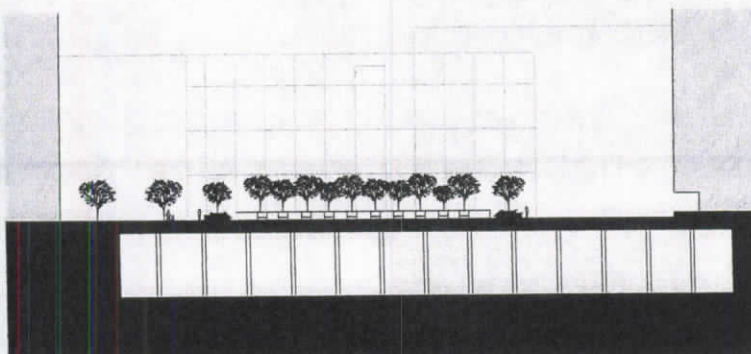
Coupe mettant en évidence l'importance du vide sous la place Jean Rey
