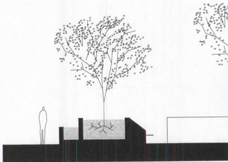
Coupe sur les bacs à plantes
