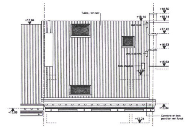
Façade avant Situation existante INCHANGÉE
