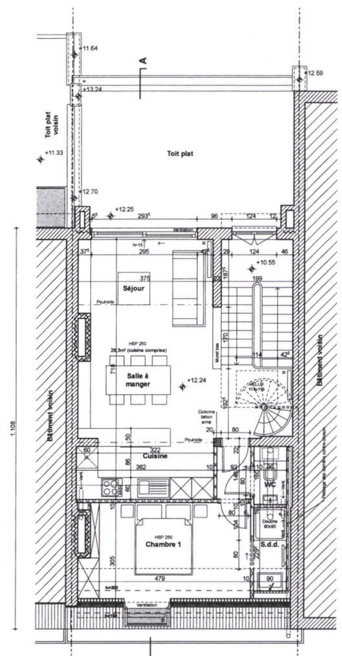
Plan du 3ème étage Situation existante
