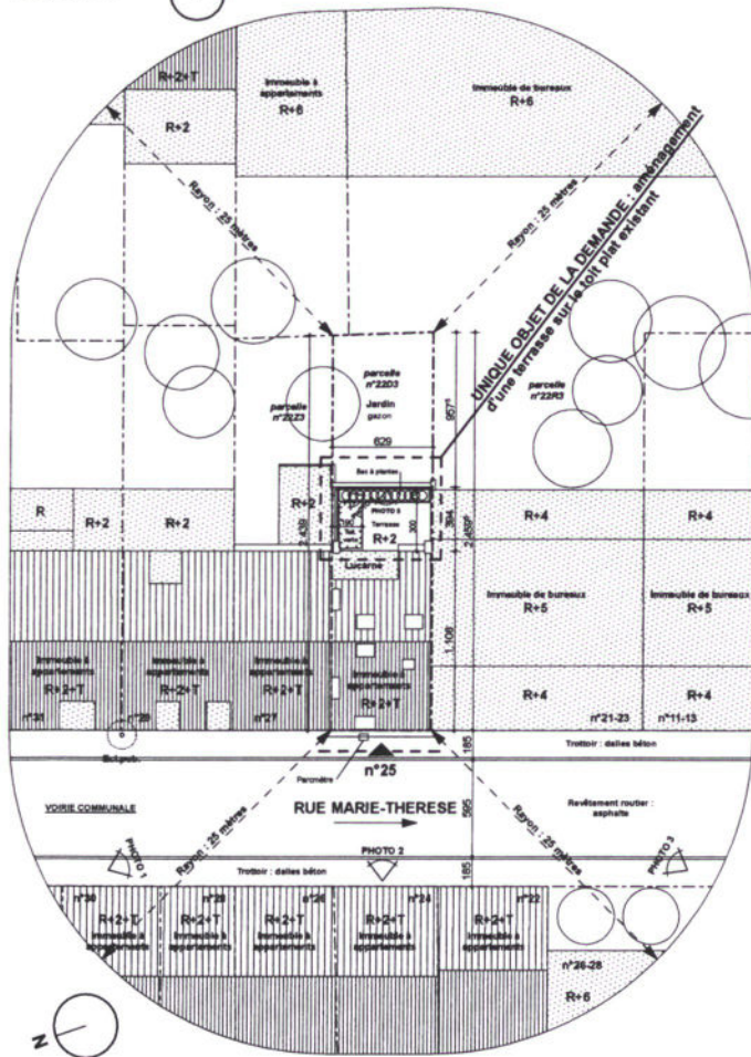
Plan d'implantation - TYPE C Ech.: 1-200
