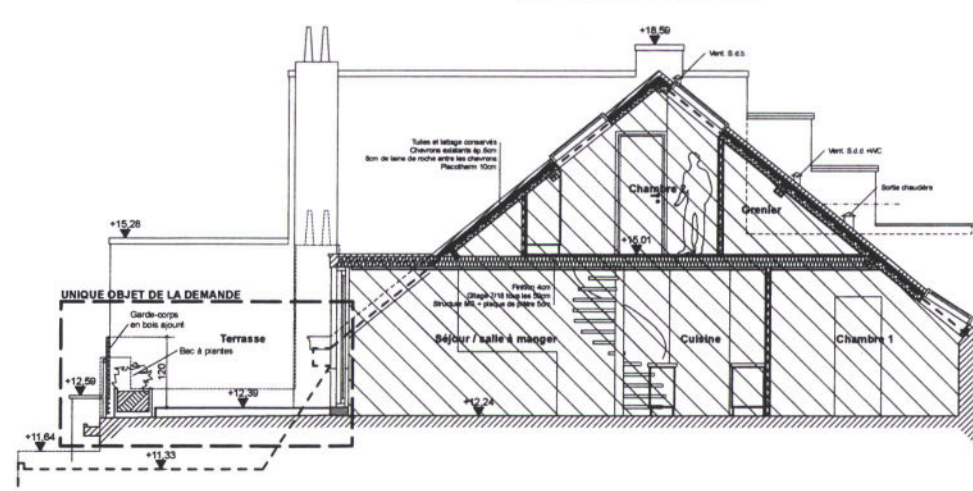
Coupe AA Situation projetée
