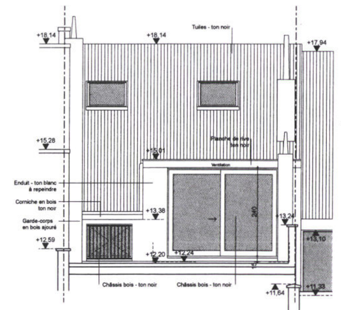
Façade arrière Situation existante
