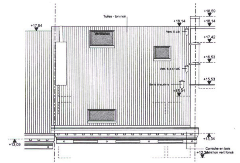
Façade avant Situation existante
