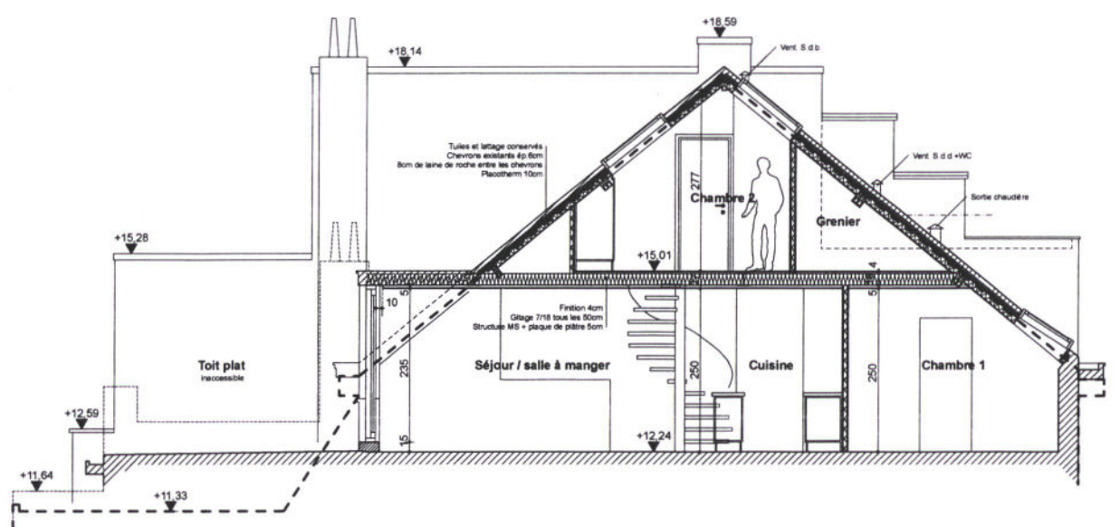
Coupe AA Situation existante
