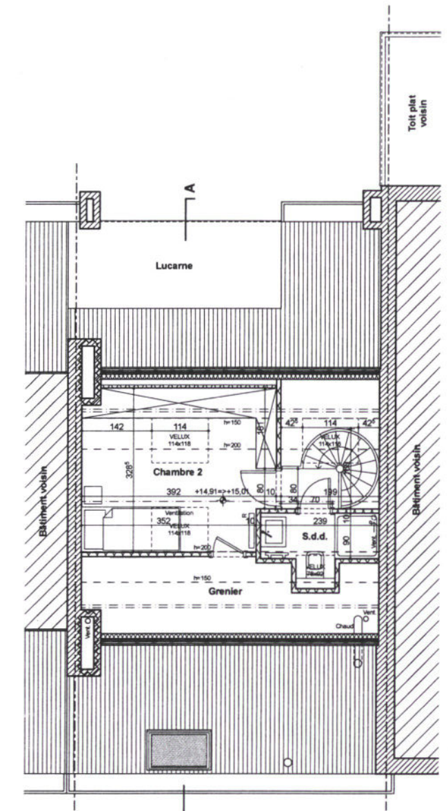
Plan des combles Situation existante
