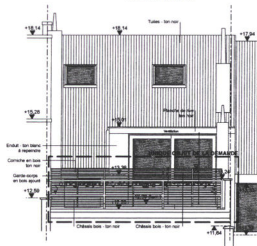
Façade arrière Situation projetée
