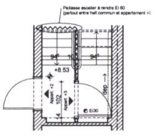
Palier du 2ème étage Situation existante
