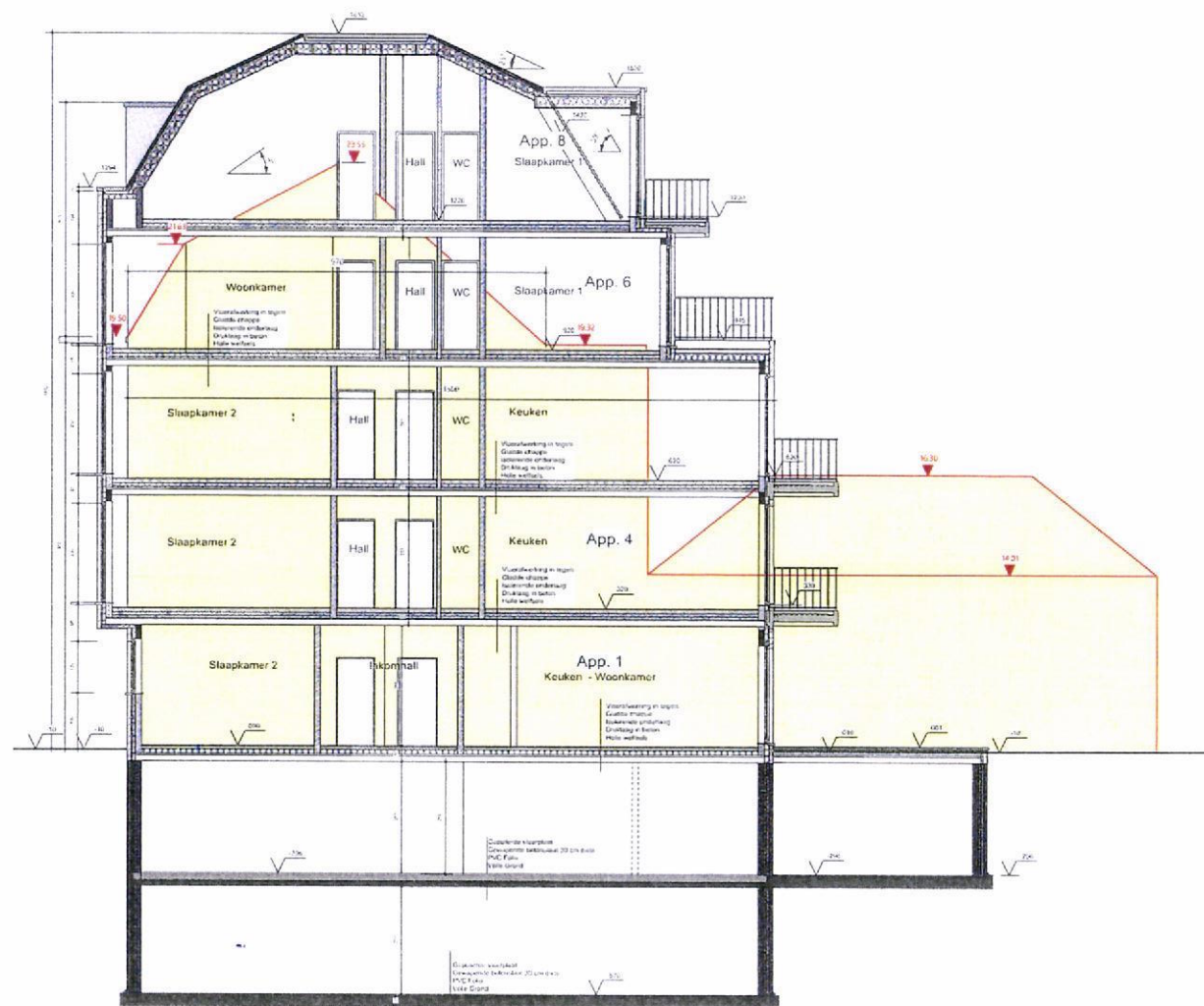
Doorsnede B - B
